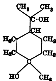
trans-Terpin.
